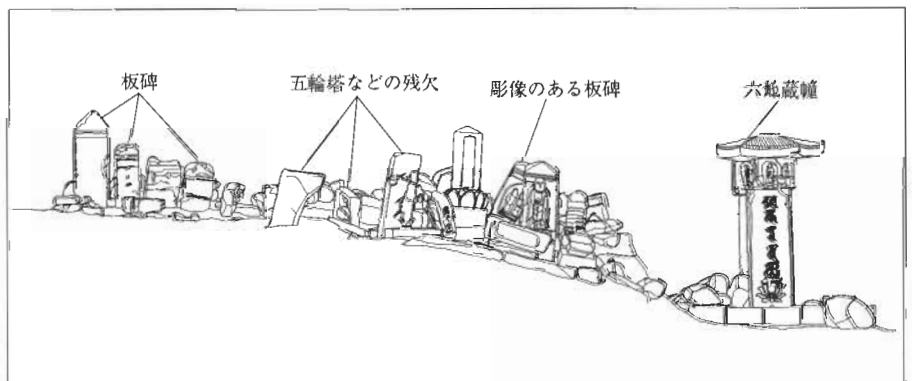
石塔群立面実測図（S=1/80）
